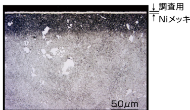
DC53マイクロ組織(窒化層50μm狙い) 化合物層なく、約50μm窒化層 断面硬さ分布:図DC53を参照
