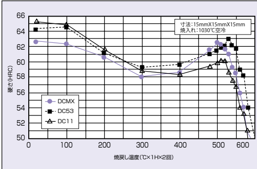
■ 焼入焼戻し曲線
