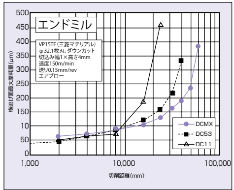
■ 被削性(焼なまし)
